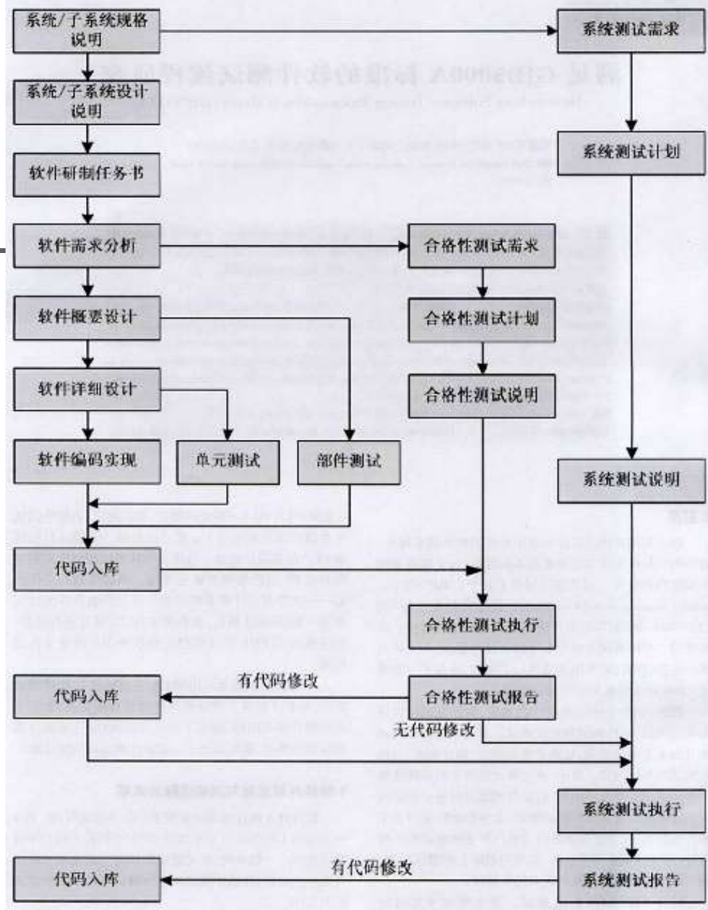
软件测试过程与开发过程并行示意图
